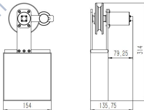
图3-4 ZKXG100-S尺寸
