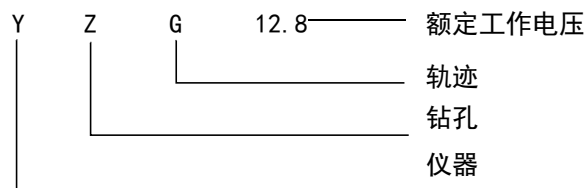
图1-1 型号示意图
