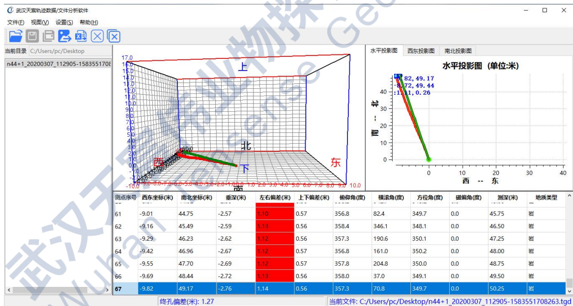
图3-11 轨迹对比图
