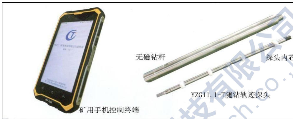
图1-2 装置结构分解图
