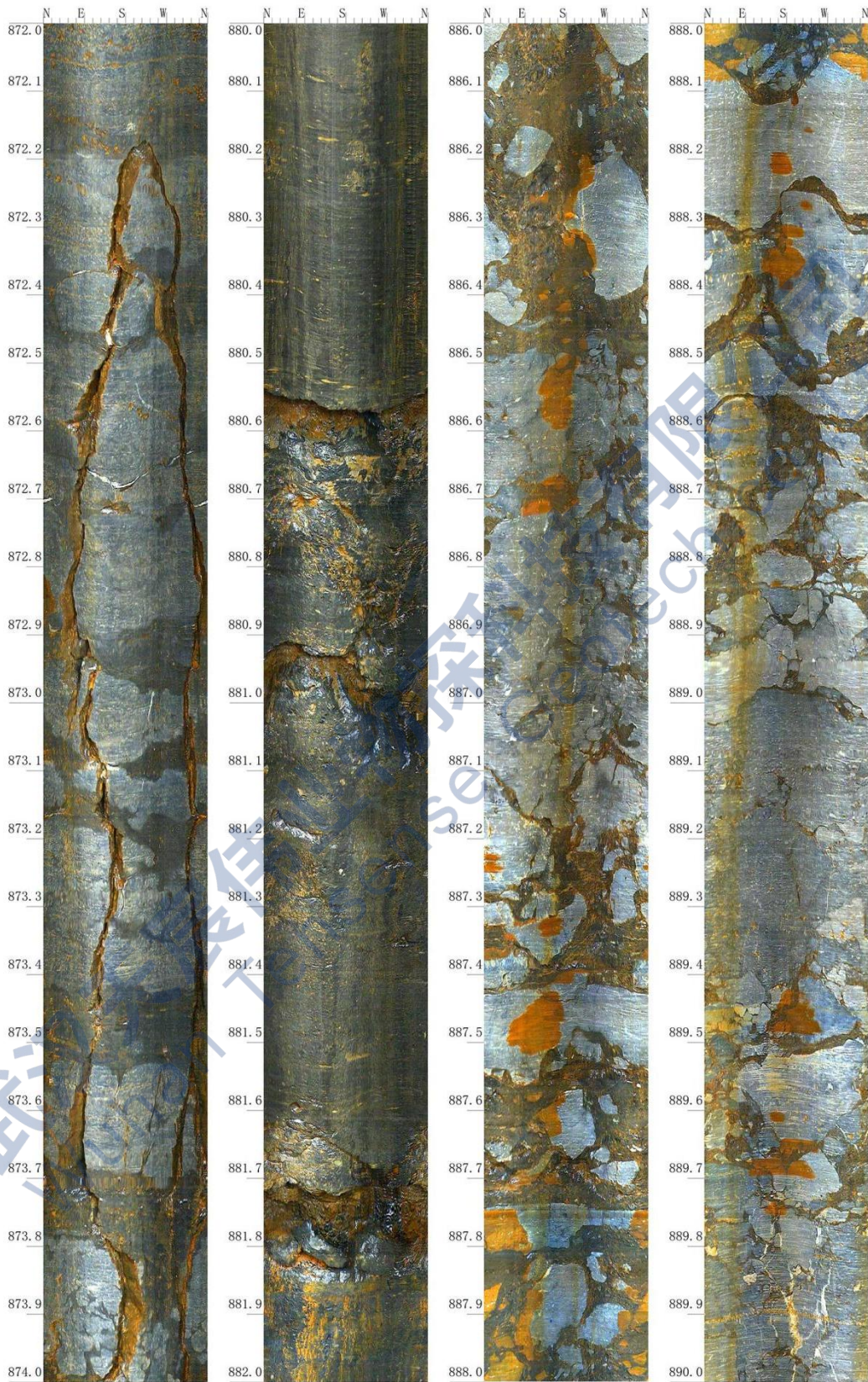
平面展开图
